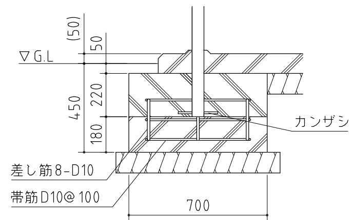
A-A' 断面 1/20
